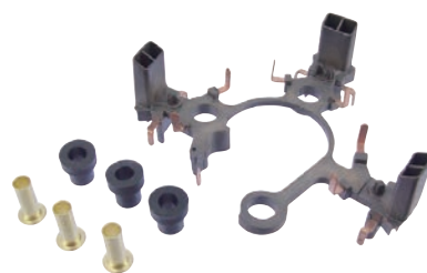
31-82501 Repair Kit-Rectifier
