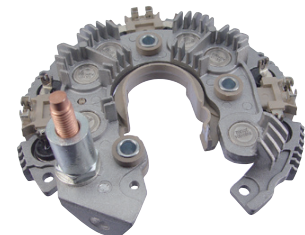
31-82046 Rectifier 134mm OD
