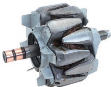
30-82036 Rotor 128.7 mm OD 200 Amp
